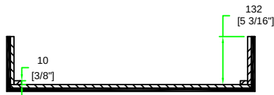
A-A VIEW
