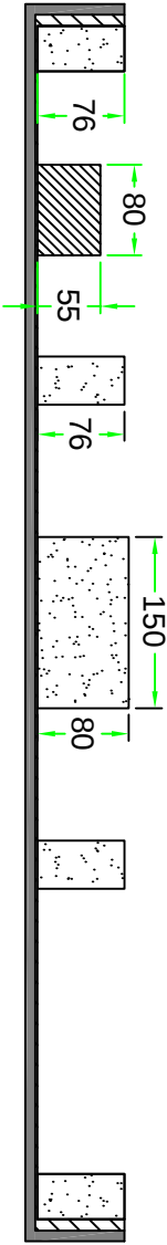
A-A VIEW
