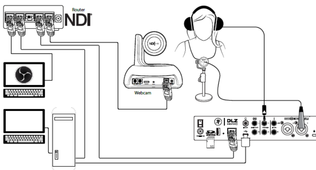
接続図 3 – デュアルボックス構成
