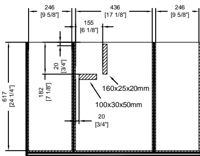
A-A View
