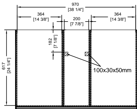
A-A View
